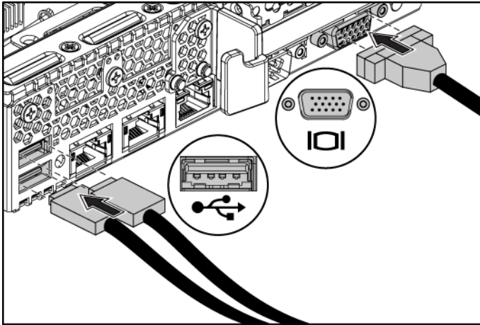
Abbildung 4. Optional – Anschließen von Tastatur, Maus und Bildschirm
