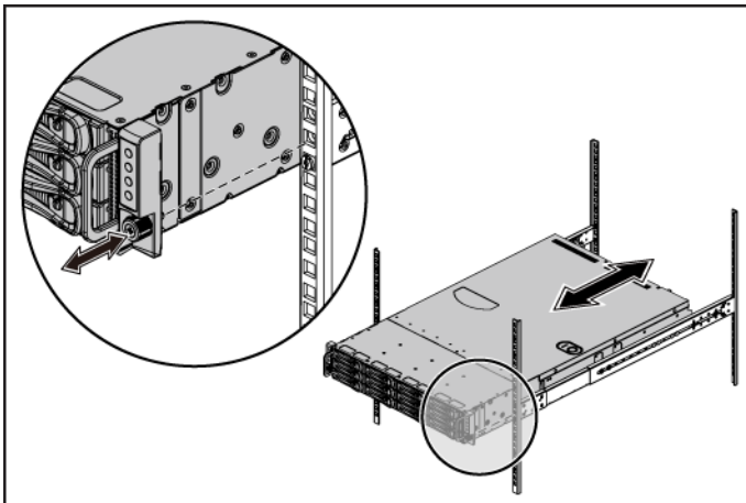
Abbildung 3. Installieren des Gehäuses im Rack.
